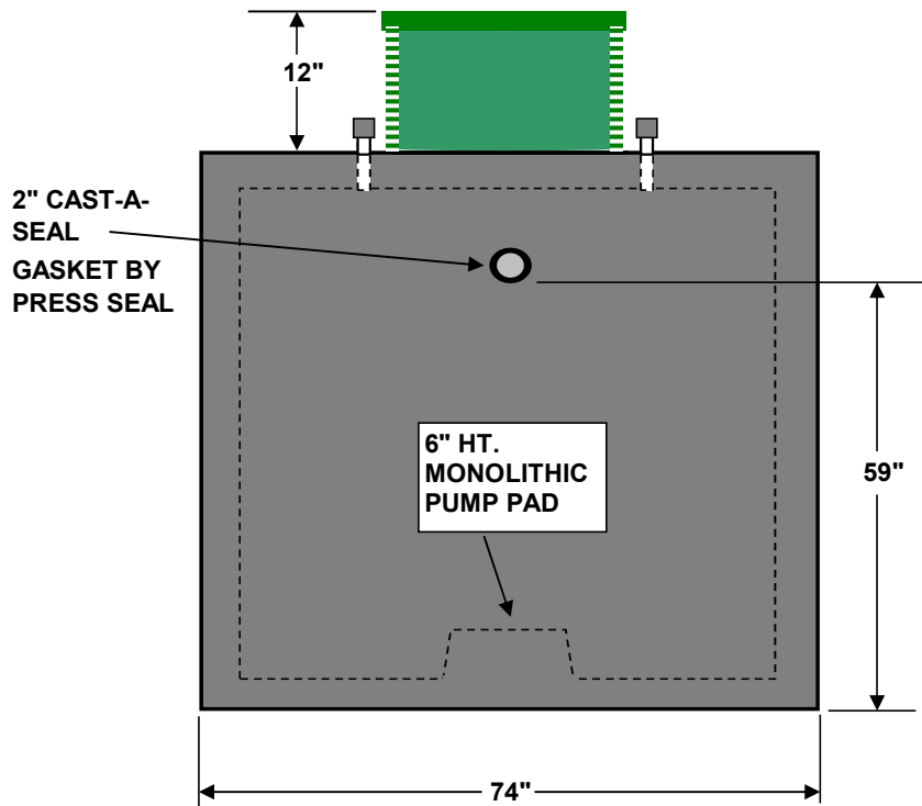
OUTLET END
